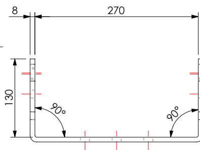
Vue latérale :
