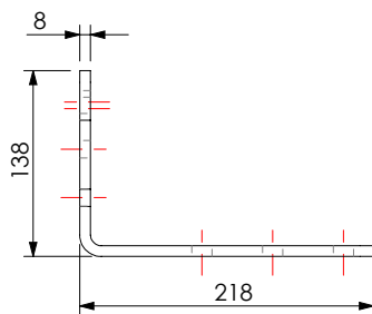
Seitenansicht:
