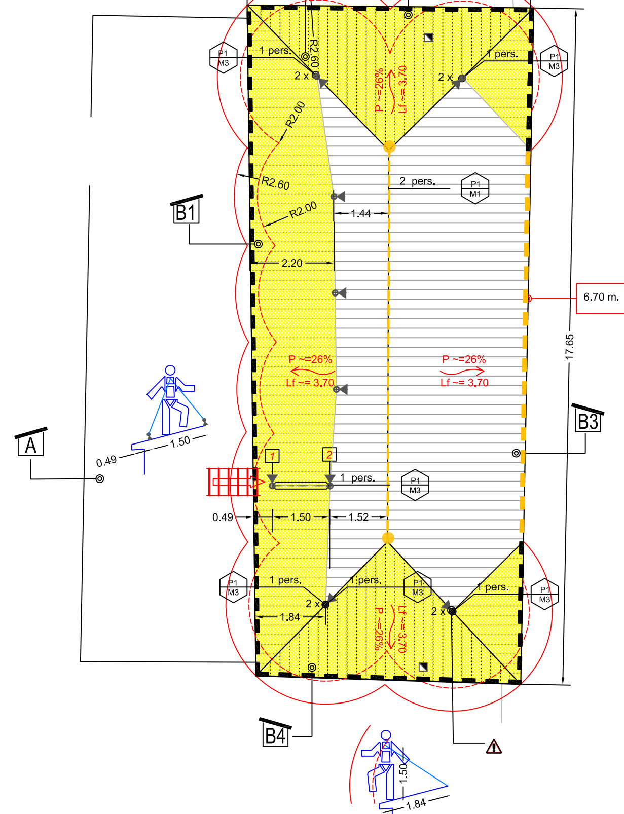
Pianta Copertura
